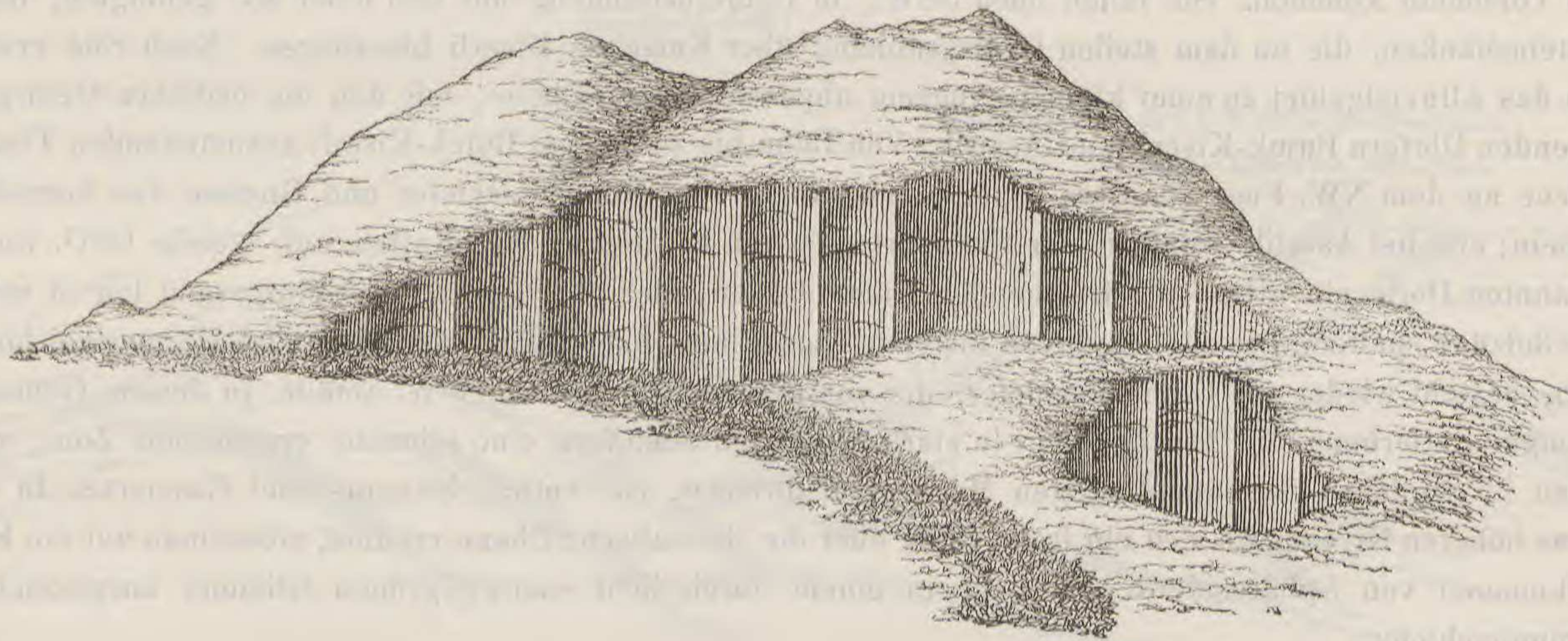
Fig. 6. Künstlicher Aufschluss in den Serpentinbreccien von Karatschair.
